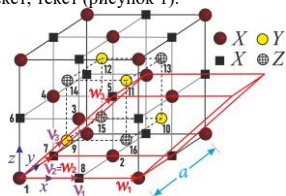
Рисунок 1 – Вектора напряженности электростатического поля двух атомов
